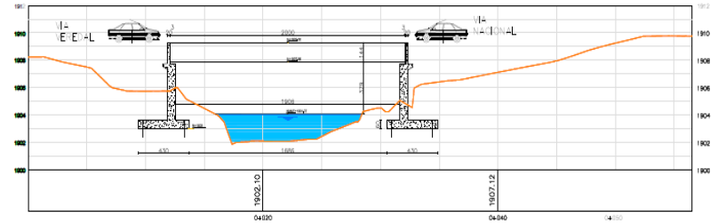
PERFIL PUNTE NUEVO SAN JOAQUIN ESCALA 1:100
